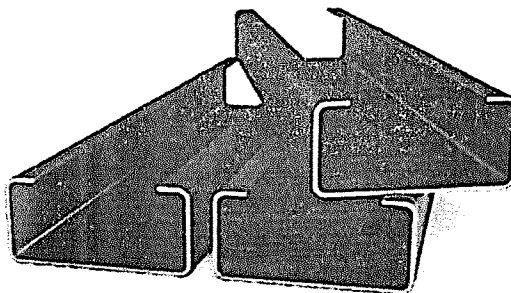
Imagem 5: Perfil U enrijecido.
